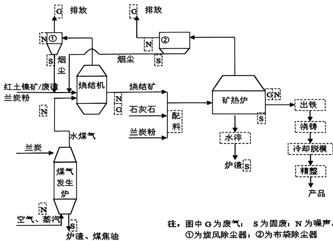
生产工艺流程及产污环节图
