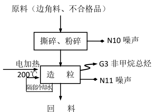
图 2-5 回料生产工艺流程及产污环节图
