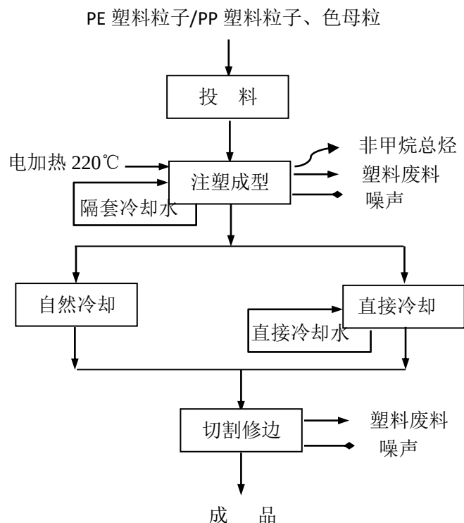
图 2-5 现有项目塑料管材生产工艺流程及产污环节图
