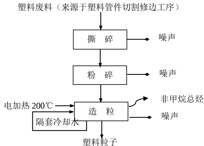
图 2-6 现有项目废料回收造粒生产工艺流程及产污环节图
