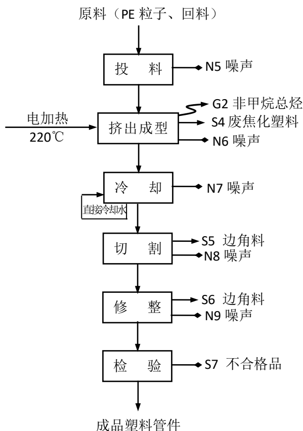
图 2-4 塑料管材生产工艺流程及产污环节图
