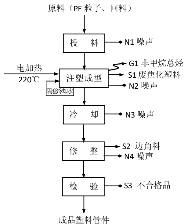
图 2-3 塑料管件生产工艺流程及产污环节图
